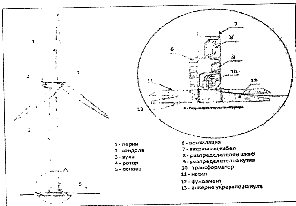
Фиг.№3. Индикативна схема на вятърна турбина
